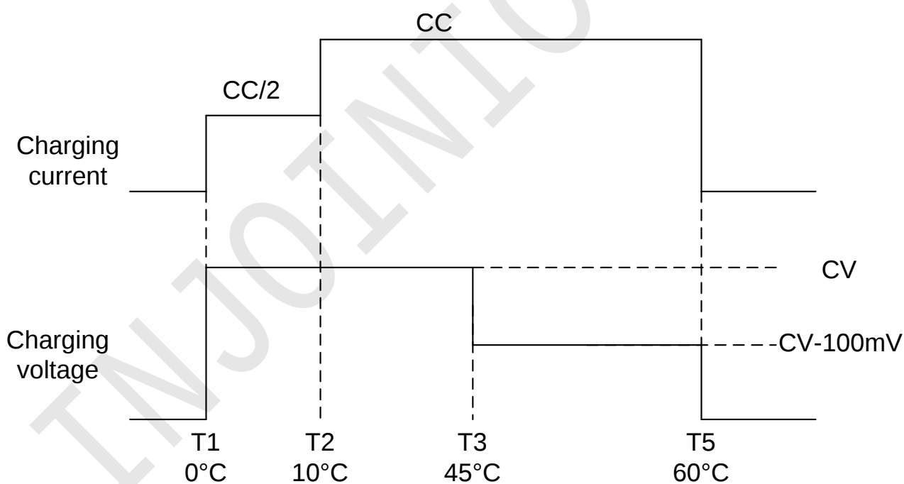
图 10 5 段式电池温度充电保护（兼容 JEITA 标准）示意图
