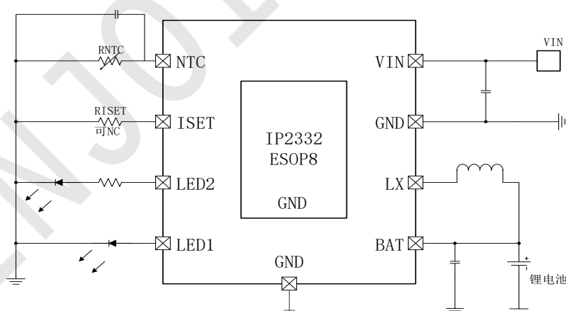
图 1 简化应用原理图
